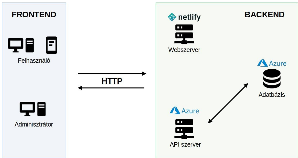
5.1. ábra. A rendszer architektúra diagramja
