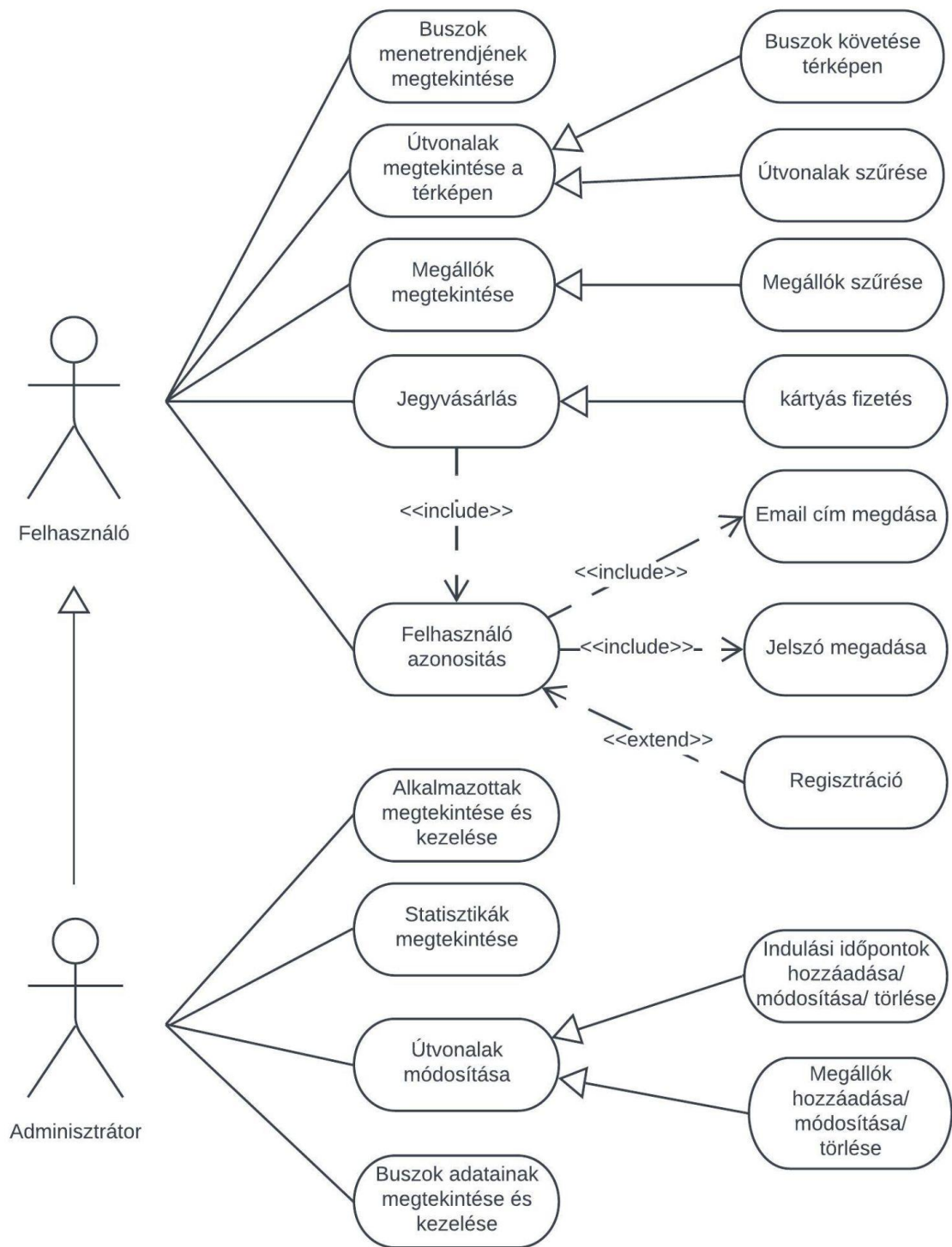
4.1. ábra. Use-case diagram a felhasználók és az adminisztrátorok lehetőségeiről
