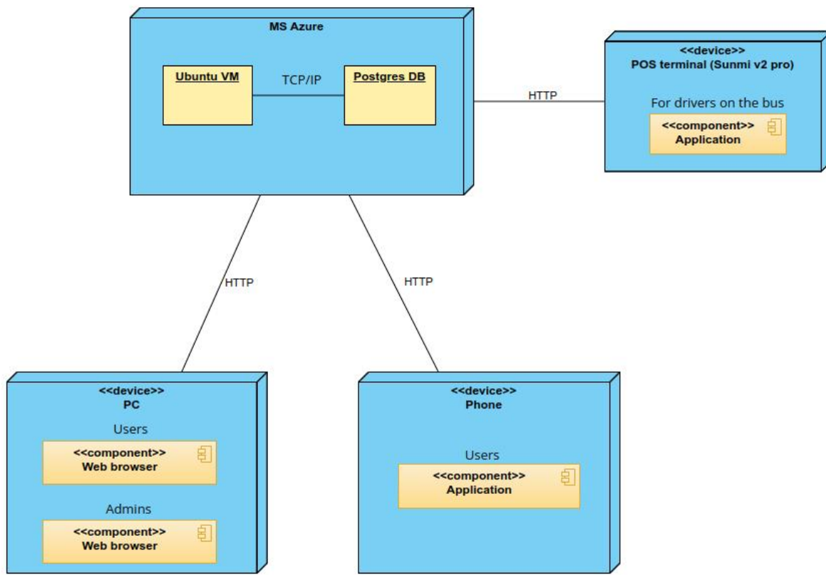
6.1. ábra. Telepítési diagram
